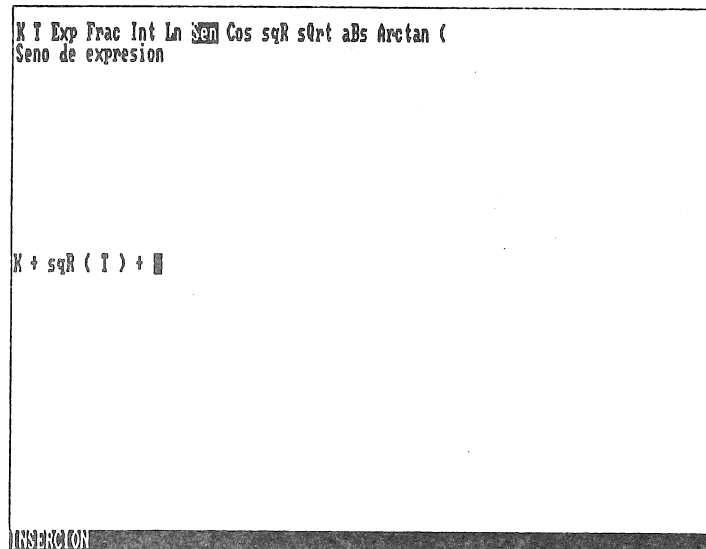
Figura 2. Especificación de una función
