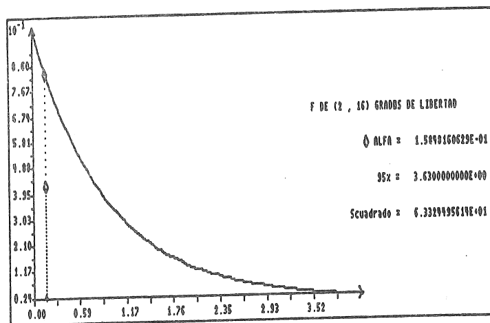
Figura 30. Estadísticos asociados a \lambda(k_2) y S(k_2)
