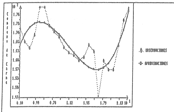
Figura 10. Resultado gráfico del modelo tendencias polinómicas
