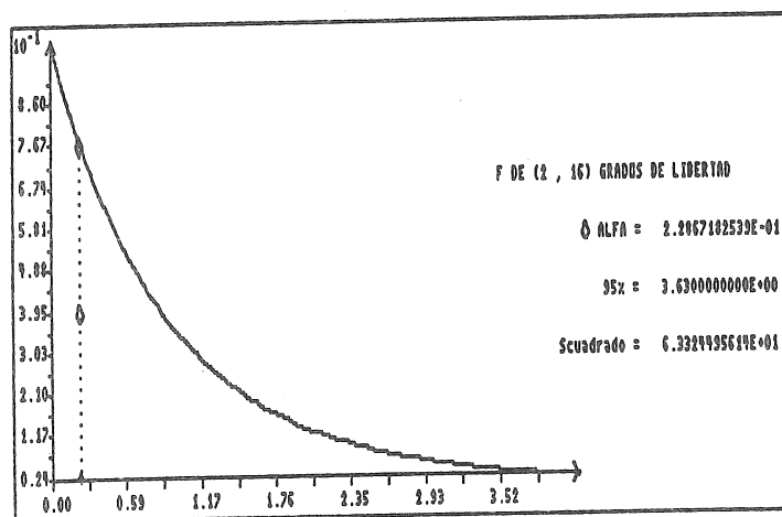
Figura 31. Estadísticos asociados a \lambda(k_3) y S(k_3)
