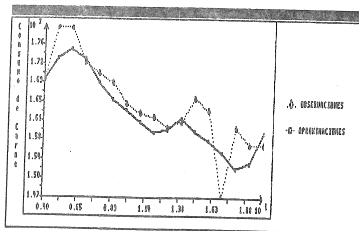
Figura 21. Resultado gráfico modelo suavizamiento
